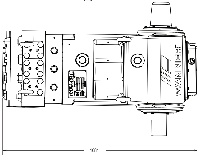
上面
