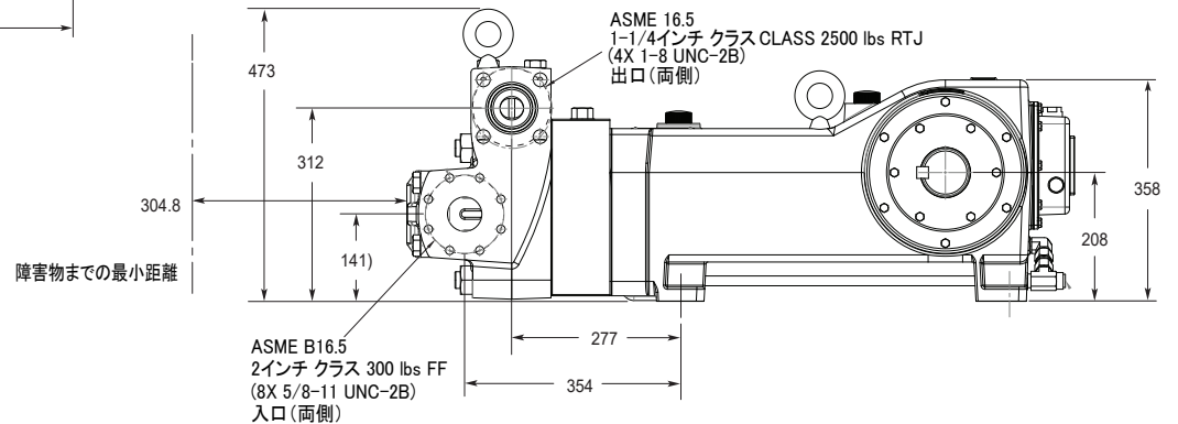
側面
