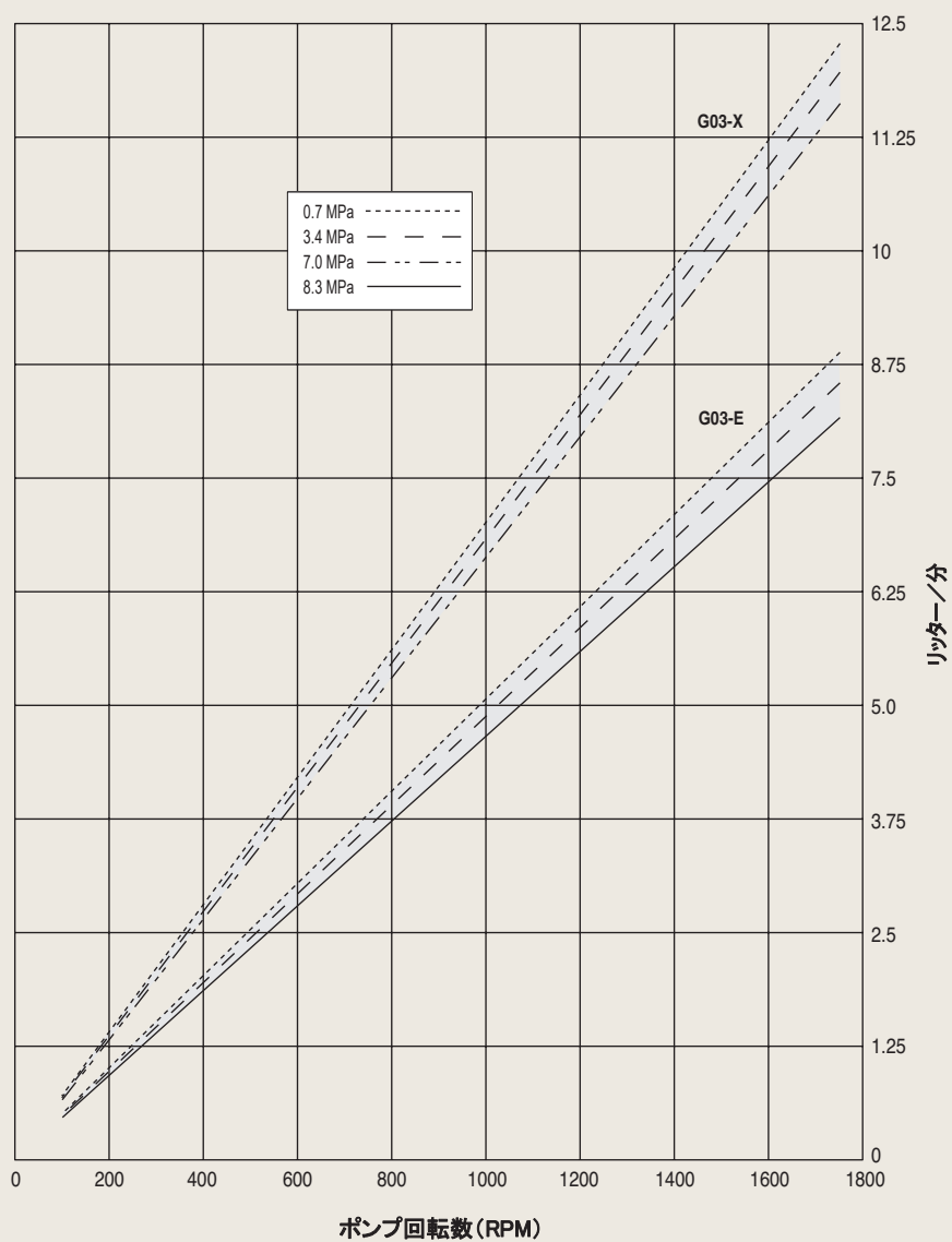
性能曲線
