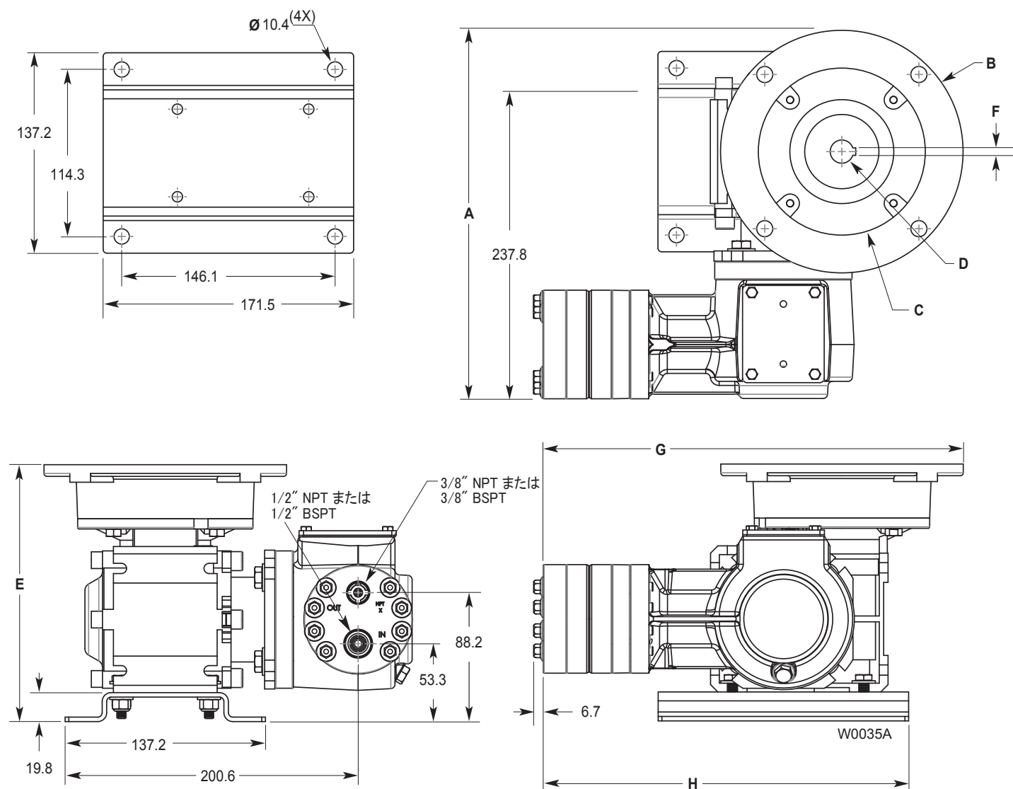
寸法図 (mm)
