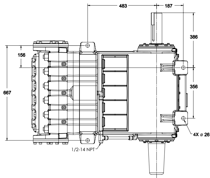
底面
